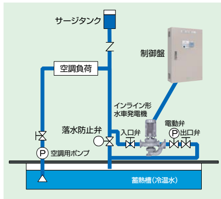
9kW 発電機
