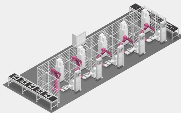
複数ロボットセルによる溶接ライン
