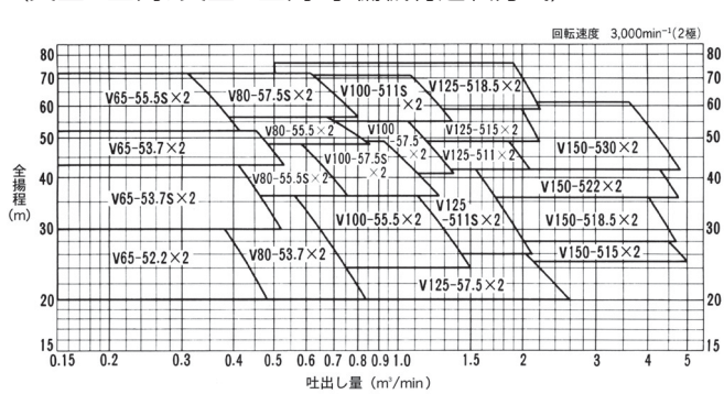
<交互+並列、交互+並列・予備機付運転方式>
