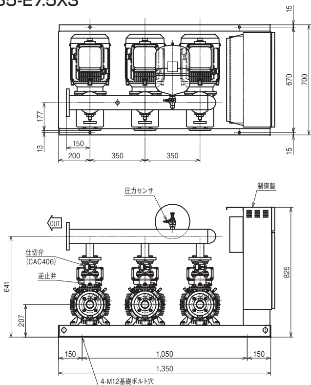
3台台数制御 (例) IJ2 65-E7.5X3
