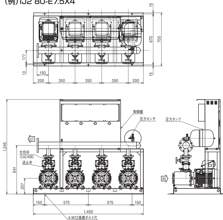
4台台数制御 (例) IJ2 80-E7.5X4
