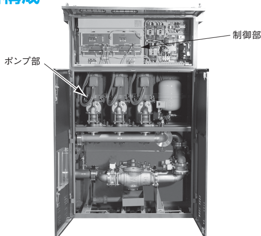
2台並列・3台ローテーション運転
