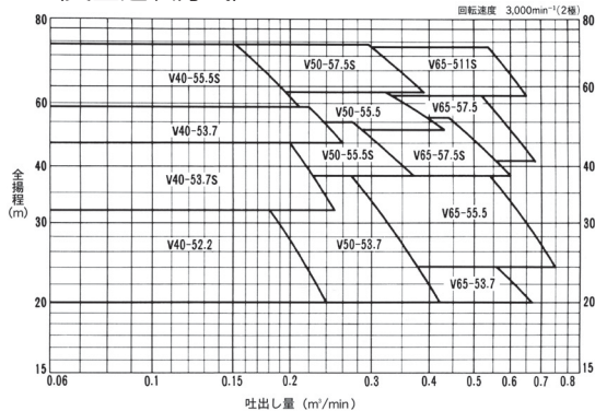
<交互運転方式>
