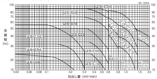
● 交互+並列運転方式
