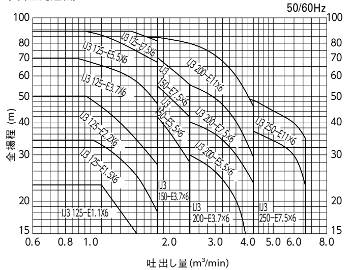
(6台並列運転)
