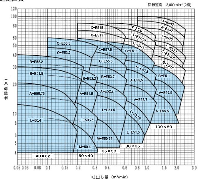
JC2形うず巻ポンプ
