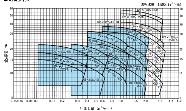
JOV2形うず巻ポンプ
