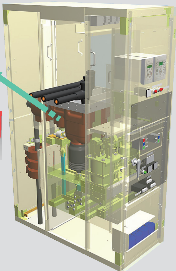
図. 二点切り三位置形真空スイッチ
