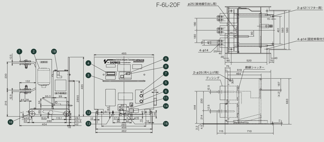
■遮断器外形寸法図
