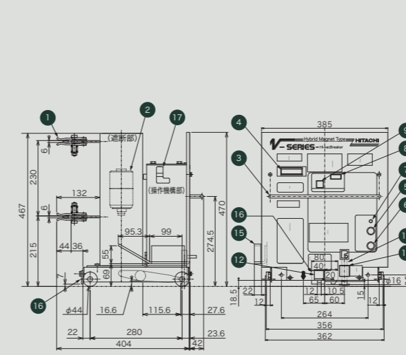
■遮断器外形寸法図
