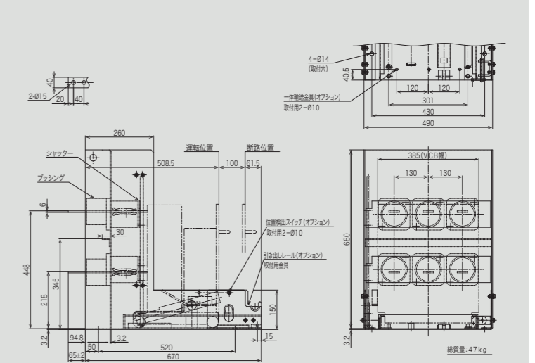
■遮断器固定枠外形寸法図
