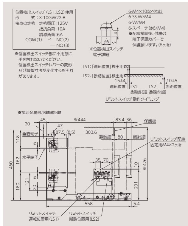
位置検出スイッチレバー
