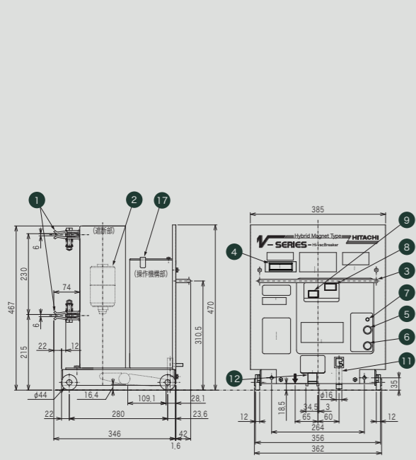
■遮断器外形寸法図
