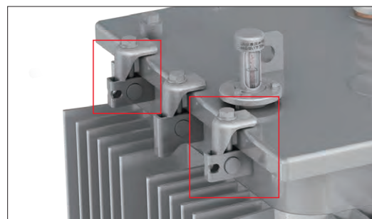
相対変位抑制用固定座(標準付属品)
